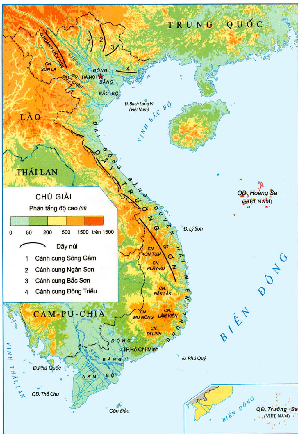
Hình 1. Lược đồ địa hình Việt Nam
