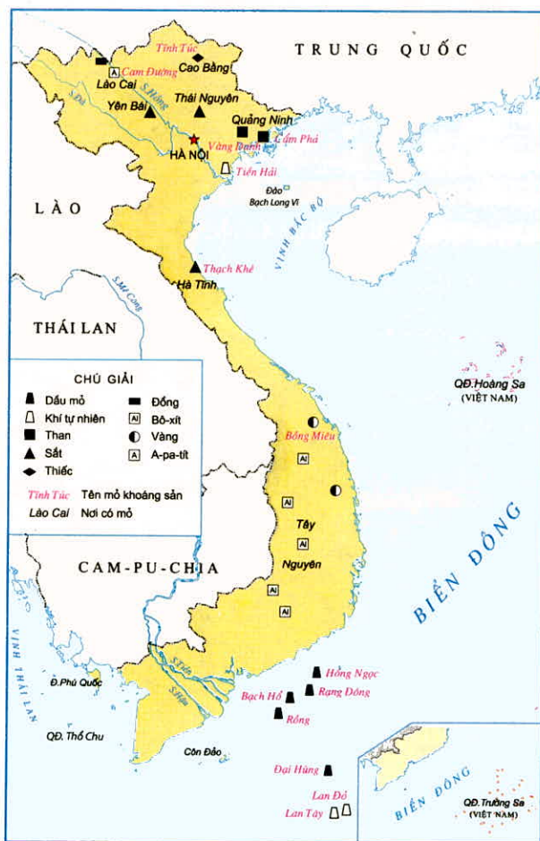
Hình 2. Lược đồ một số khoáng sản Việt Nam
